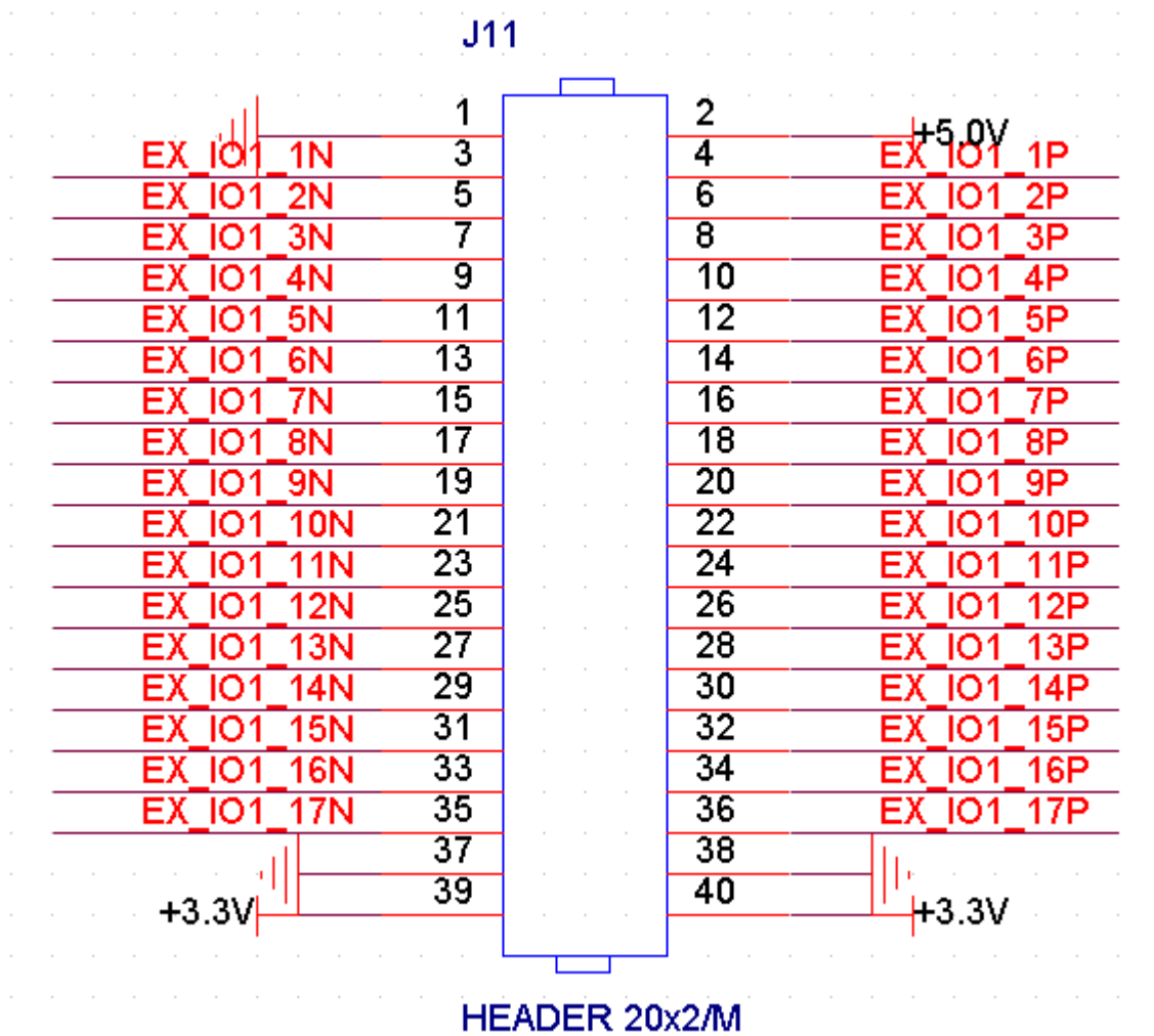
图 3-11-1 扩展口 J11 原理图
