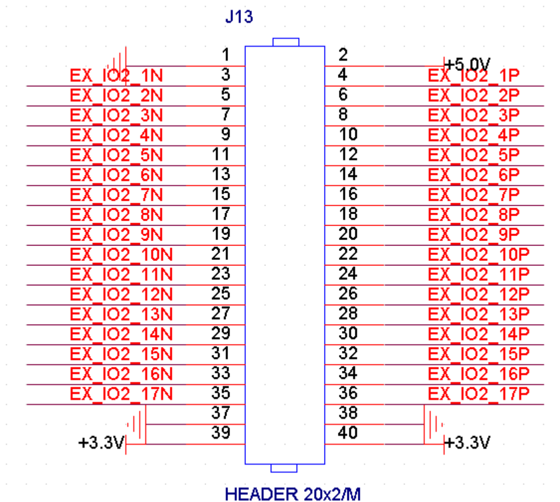
图 3-11-3 扩展口 J13 原理图
