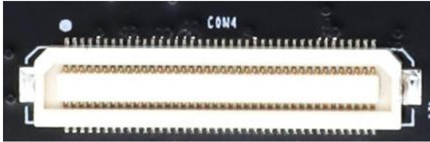
图 2-10-4 CON4 扩展口连接器的实物图
