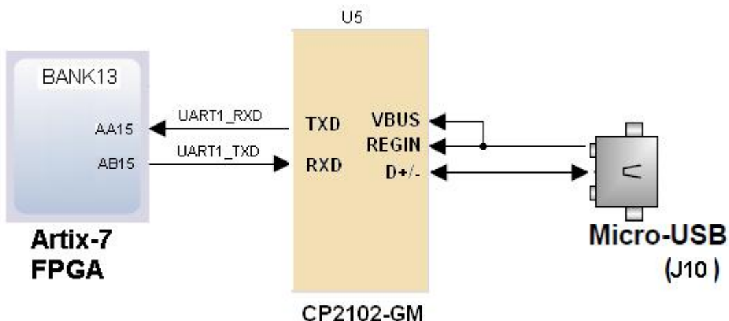
图 3-5-1 USB 转串口示意图
