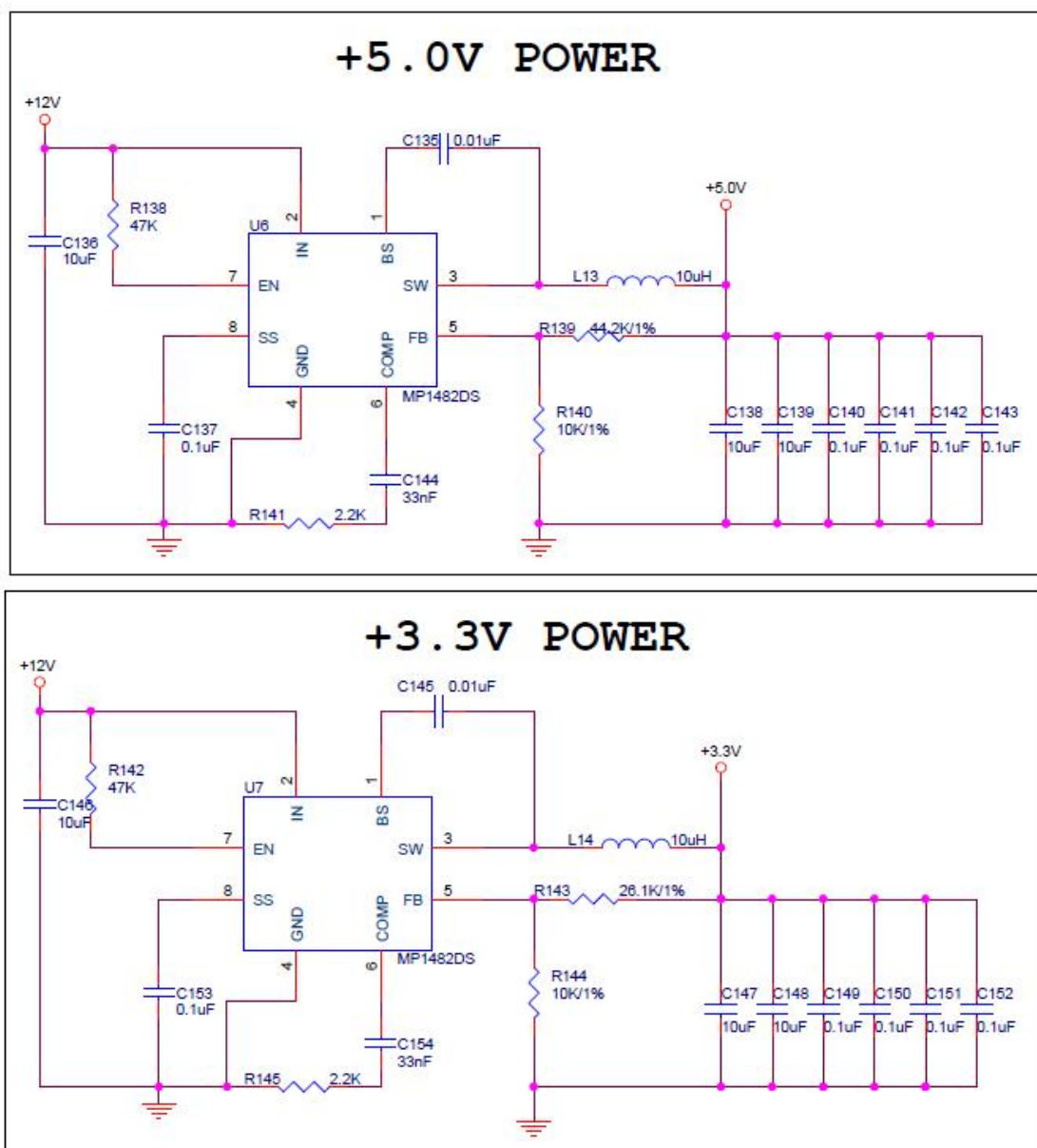
图 3-10-1 扩展板电源原理图
