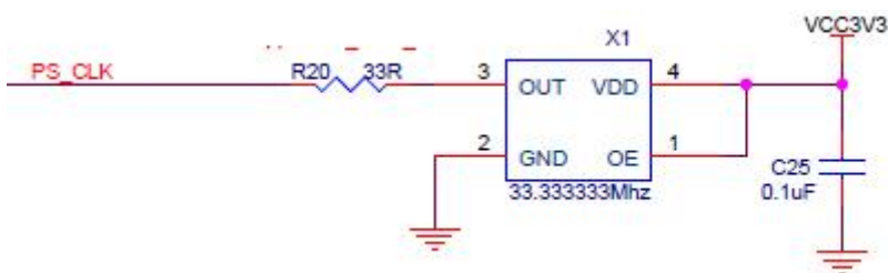
图 2-5-1 PS 部分的有源晶振
