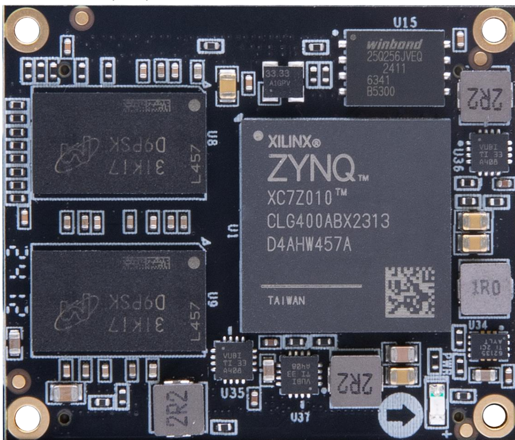
AC7Z010 核心板正面图
