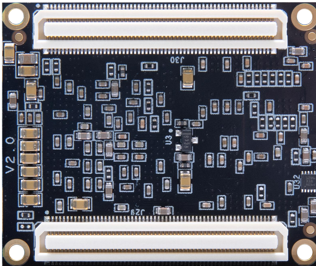
AC7Z010 核心板背面图
