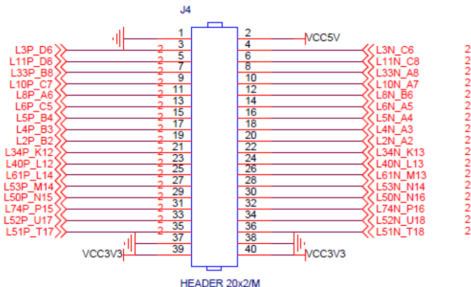
图 8.2 J4 扩展口原理图
