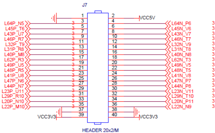
图 8.4 J7 扩展口原理图
