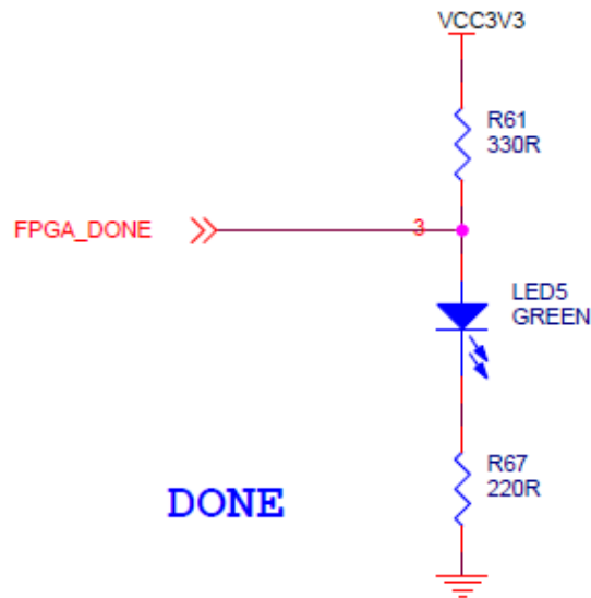
图 9.2 配置 LED 原理图
