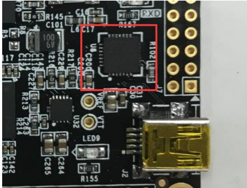
图 7.2 USB 转串口实物图
