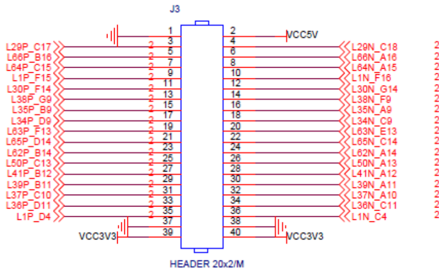
图 8.1 J3 扩展口原理图
