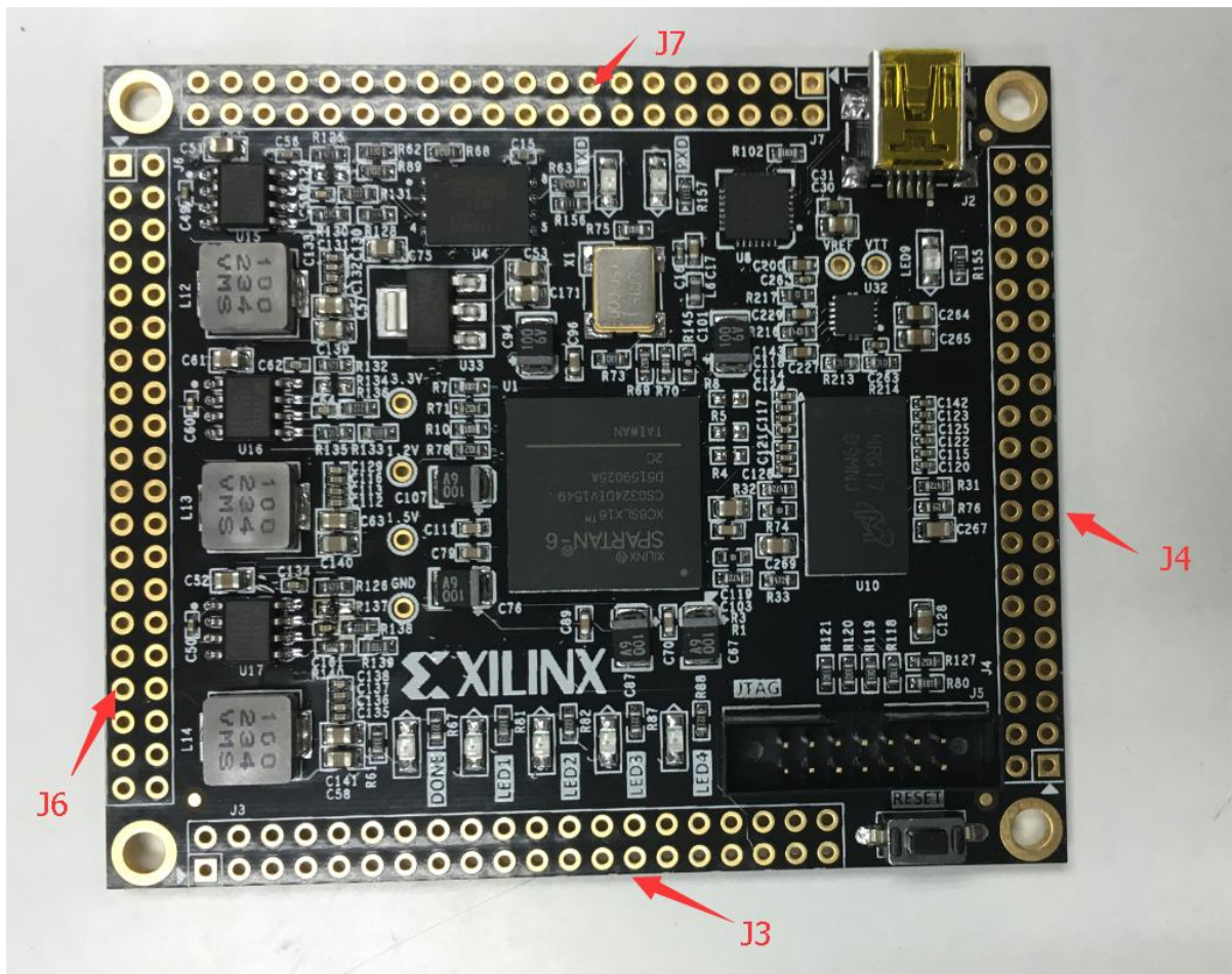
图 8.5 扩展口实物图
