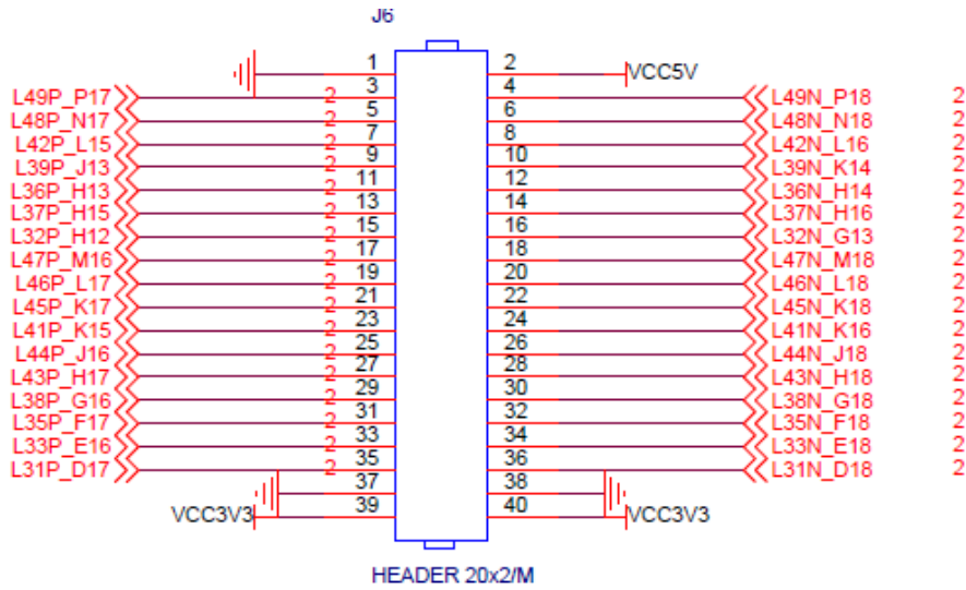
图 8.3 J6 扩展口原理图
