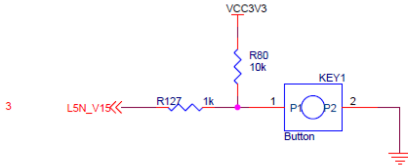
图 10.1 复位按键原理图
